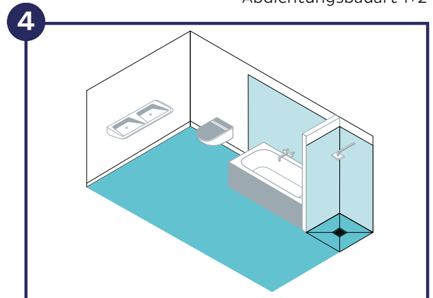
Häusliches Bad mit Badewanne ohne Brause mit bodengleicher Dusche ohne Duschartrennung Abdichtungsbauart 1+2
