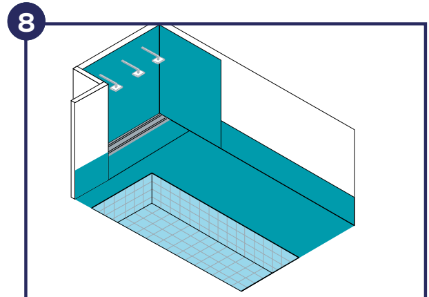
Flächen im Umgangsbereich von Schwimmbecken Abdichtungsbauart 2+3
