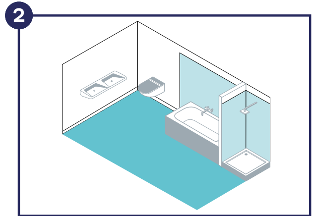
Häusliches Bad mit Badewanne ohne Brause und Duschtasse ohne Duschartrennung Abdichtungsbauart 1+2
