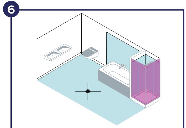
Häusliches Bad mit Badewanne ohne Brause mit Duschtasse, Duschartrennung sowie Bodenablauf im Raum Abdichtungsbauart 1+2
