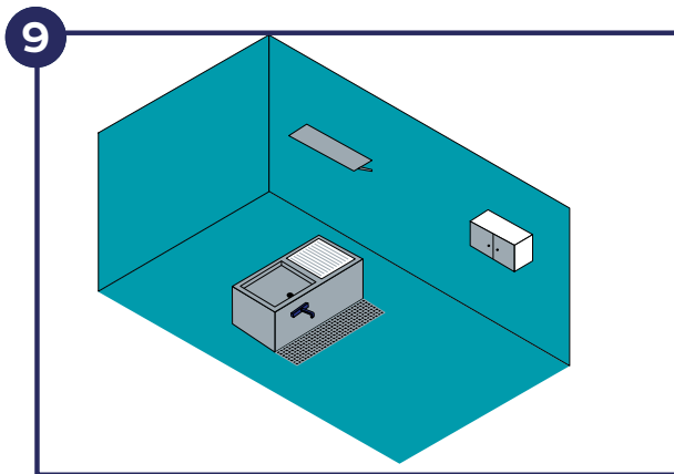
Gewerblich genutzte Großküche, ggf. mit zusätzlichen chemischen Einwirkungen Abdichtungsbauart 4
