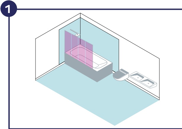
Häusliches Bad mit Badewanne, Brause und Duschartrennung Abdichtungsbauart 1+2
