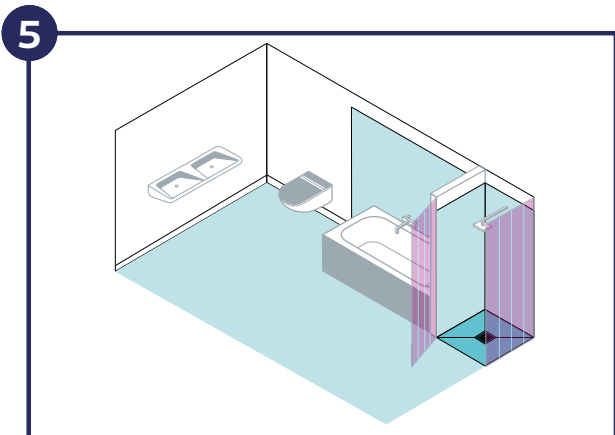
Häusliches Bad mit Badewanne ohne Brause und mit bodengleicher Dusche und Duschartrennung Abdichtungsbauart 1+2
