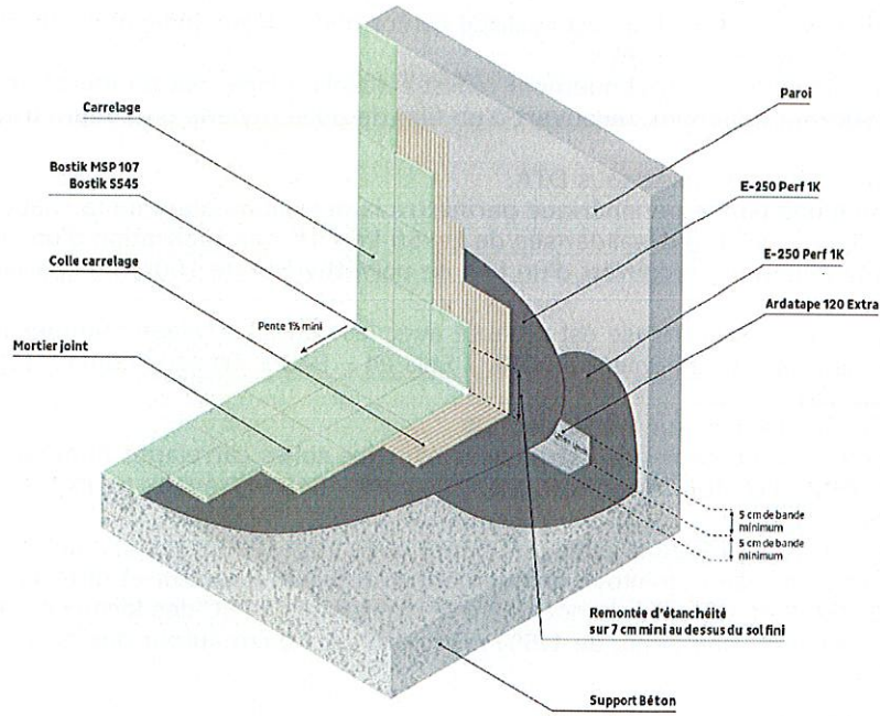
Figure 1a : Raccordement Sol / Mur en Local P3
