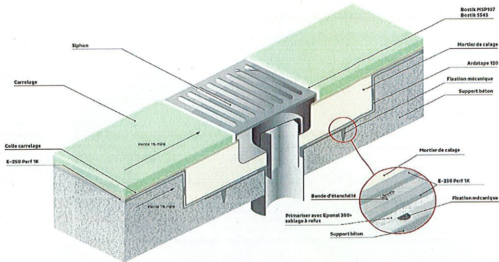
Figure 5a : Raccordement à un siphon de sol – Cas d'une pose collée d'un carrelage
