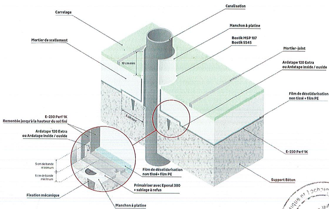
Figure 2b : Canalisation traversante en sol - cas d'une pose scellée du carrelage
