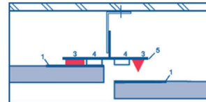
II. Stijl voor voegaansluiting - aluminium
