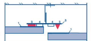
II. montant pour joints - aluminium
