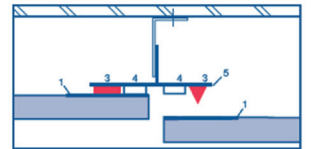
II. Montant en aluminium
