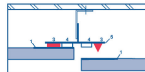
II. Montant pour les joints - aluminium
