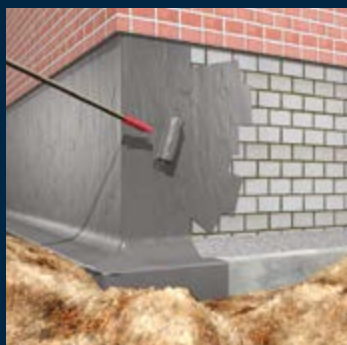
Afdichting buitenzijde Betonnen muren
